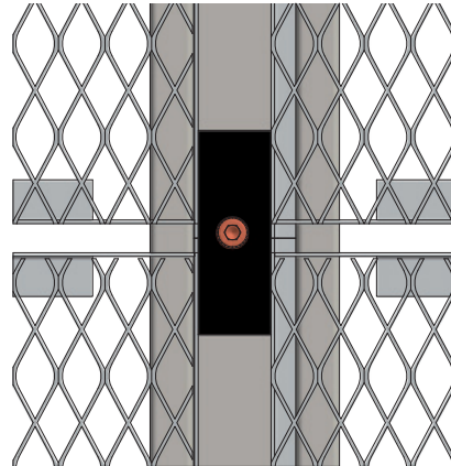
Deckenuntersicht, Kreuzungspunkt von vier Deckenplatten mit Niederhalteplatte widok dolny
