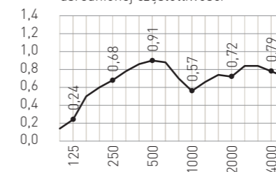
Chłonność akustyczna Współczynnik pochłaniania dźwięku w uśrednionej częstotliwości
