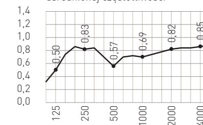
Chłonność akustyczna Współczynnik pochłaniania dźwięku w uśrednionej częstotliwości
