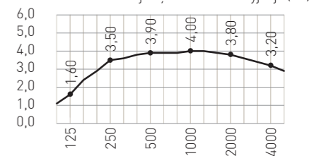
Chłoność akustyczna Powierzchnia pochłaniająca dźwięk A_{p,0} /m 2 do uśrednionej częstotliwości tercyjnej f [Hz]
