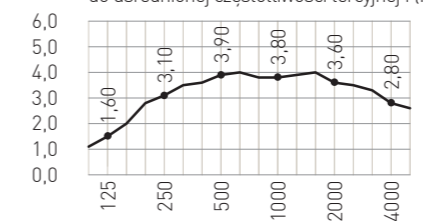
Chłoność akustyczna Powierzchnia pochłaniająca dźwięk A_{p,0} /m 2 do uśrednionej częstotliwości tercyjnej f [Hz]
