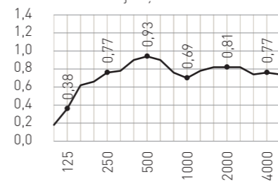
Chtonność akustyczna Współczynnik pochłaniania dźwięku w uśrednionej częstotliwości
