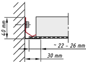
Wandanschluss für Anschnittkassetten mit L - Winkel und Niederhalteprofil (geeignet für Kassettentyp A/B/C) Attacco a parete per pannelli tagliati con angoli a L e profi- lo a clip (adatto per tipo pannelli A/B/C)
