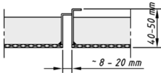
Kassettenlängsfuge mit Distanzierung (Typ A/C) Giunto longitudinale del pannello con distanziatore (tipo A/C)
