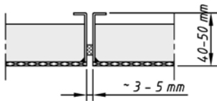
Kassettenlängsfuge mit Dichtband bei Kassetten mit stumpf aufgeschweißten Stegen (Typ A) Giunto longitudinale con guarnizione nei pannelli con risvolti saldati smussati (tipo A)
