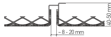
Kassettenlängsfuge mit Distanzierung (Typ B) Giunto longitudinale del pannello con distanziatore (tipo B)
