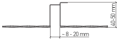
Kassettenlängsfuge mit Distanzierung (Typ A) Giunto longitudinale del pannello con distanziatore (tipo A)
