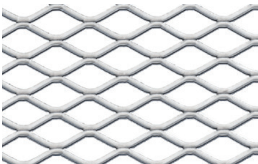
Masche Maglia freier Querschnitt ca. sezione libera ca. 66,7 %
