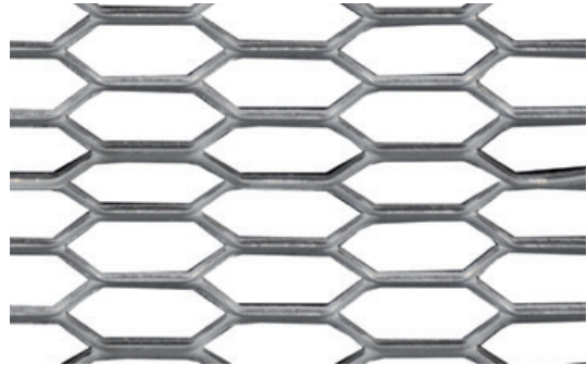
Masche Maglia freier Querschnitt ca. sezione libera ca. 44 x 10 x 2 x 1,5 [mm] 60,0%
