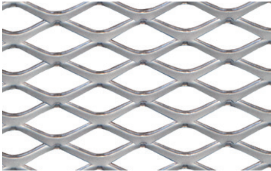
Masche Maglia freier Querschnitt ca. sezione libera ca. 30 x 15 x 4 x 1,5 [mm] 46,3%
