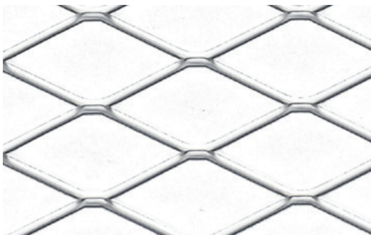
Masche Maglia freier Querschnitt ca. sezione libera ca. 50 x 22 x 2,5 x 1,5 [mm] 77,3%
