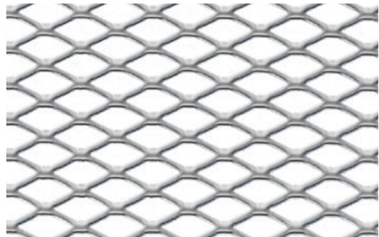
Masche Maglia freier Querschnitt ca. sezione libera ca. 62,5%
