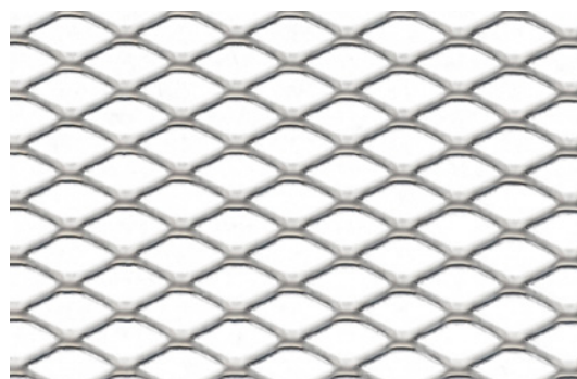
Masche 16 x 8 x 1,5 x 1,0 [mm] Maglia freier Querschnitt ca. 62,5% sezione libera ca.
