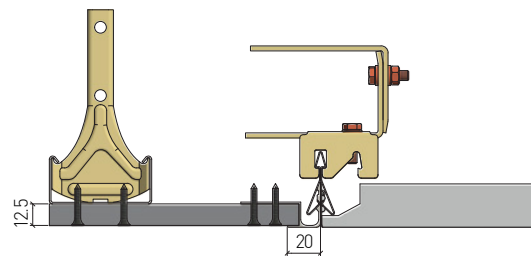
Anschluss Gipskartenfries mit Übergangsprofil GK, versetzt verschrauben Raccordement frise plaque de plâtre avec profil de transition GK, visser en quinconce
