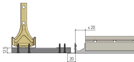
Anschluss Kassetten an der Feldstirnseite an Gipskartenfries mit Übergangsprofil GK, versetzt verschrauben Raccordement cassettes face frontale du champ à la frise plaque de plâtre avec profil de transition GK, visser en quinconce.
