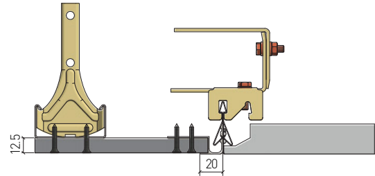
Anschluss Gipskartenfries mit Übergangsprofil GK, versetzt verschrauben
