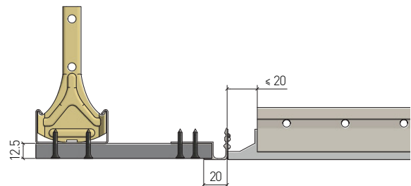
Anschluss Kassetten an der Feldstirnseite an Gipskartenfries mit Übergangsprofil GK, versetzt verschrauben
