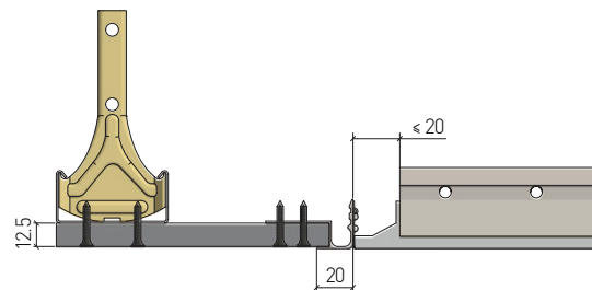
Anschluss Kassetten an der Feldstirnseite an Gipskartonfries mit Übergangsprofil GK, versetzt verschrauben Attacco pannelli sulla parte frontale del cartongesso con profilo di raccordo GK, avvitare in modo sfalsato.
