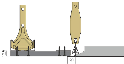
Anschluss Gipskartonfries mit Übergangsprofil GK, versetzt verschrauben Attacco cartongesso con profilo di raccordo GK, avvitare in modo sfalsato.
