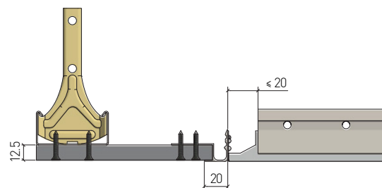
Anschluss Kassetten an der Feldstirnseite an Gipskartonfriese mit Übergangsprofil GK, versetzt verschrauben Raccordement cassettes face frontale du champ à la frise plaque de plâtre avec profil de transition GK, visser en quinconce.
