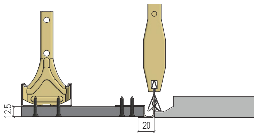
Anschluss Gipskartonfriese mit Übergangsprofil GK, versetzt verschrauben Raccordement frise plaque de plâtre avec profil de transition GK, visser en quinconce
