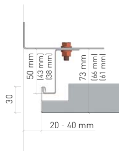
Abschluss für ganze Kassette mit Z-Einhängeprofil Pose cassette entière sur profil Z
