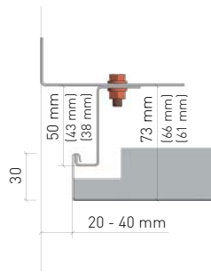
Abschluss für ganze Kassette mit Z-Einhängesprofil Wall connection for entire tile with hang-in rail
