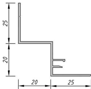
Schattenfederleiste 20/20 Profil à joint creux 20/20 pour clips
