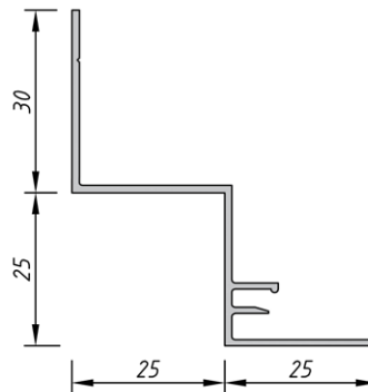
Schattenfederleiste 25/25 Profil à joint creux 25/25 pour clips
