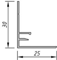
Federleiste 30/25 Profil mural pour clips 30/25
