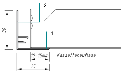
Auflage für ganze Kassette Pose cassette entière
