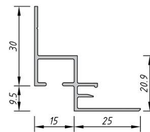
Bilderschiene 15/10 Cornière à cimaise 15/10
