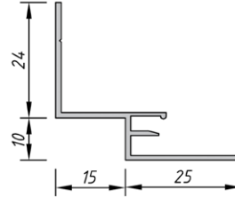
Schattenfederleiste 15/10 Profil à joint creux 15/10 pour clips
