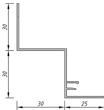
Schattenfederleiste 30/30 Profil à joint creux 30/30 pour clips
