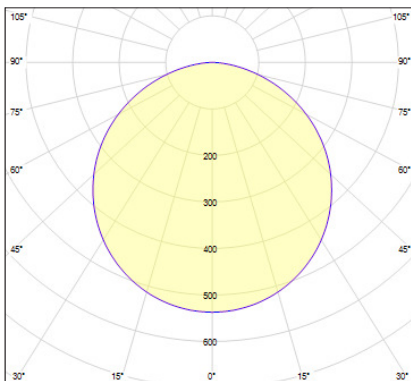
Lichtverteilungskurve (Daten auf Anfrage) Light distribution curve (data on request)
