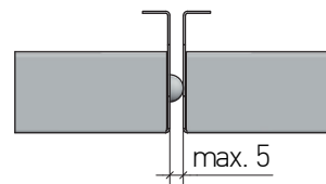
Distanzprägung Distance embossing
