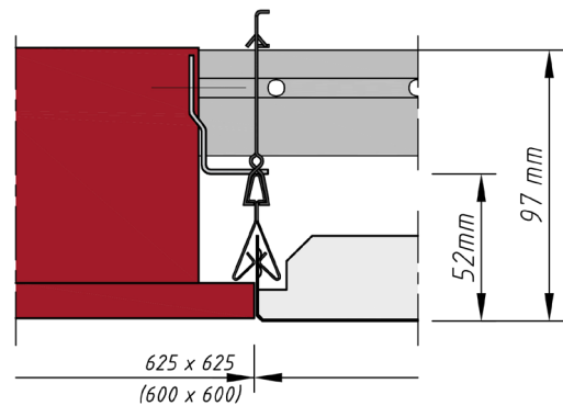
Schnitt: Leuchte / Rostprofil Doorsnede: Armatuur / Klemprofiel
