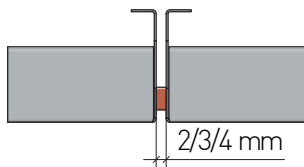
Dichtband taśma uszczelniająca
