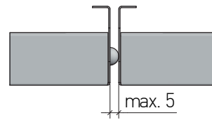
Distanzprägung Wytłoczenie dystansowe
