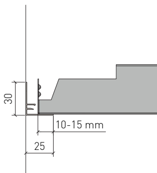
Auflage für ganze Kassette Nakładanie całego kasetonu
