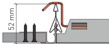
Anschluss Gipskartonfries Przyłączenie z fryzem gipsowo-kartonowym
