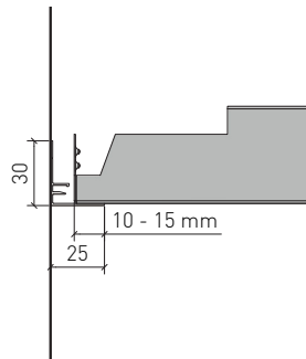
Auflage für ganze Kassette Nakładanie całego kasetonu
