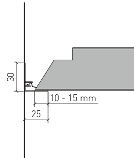
Auflage für Kassette Nakładanie dociętego kasetonu
