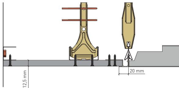
Stirnseitiger Anschluss an GK-Fries mit Übergangprofil GK (Art. Nr. 3080047 RAL 9010), Profil versetzt verschrauben. Przyłączenie kasetonu po stronie czołowej sufitu z fryzem gipsowo-kartonowym z profilem łączącym GK (nr art. 3080047 RAL 9010), profil przykręcany naprzemiennie
