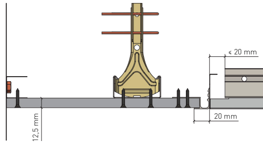
Längsseitiger Anschluss an GK-Fries, Profil versetzt verschrauben. Przyłączenie kasetonu po stronie czołowej sufitu z fryzem gipsowo-kartonowym, profil przykręcany naprzemiennie.
