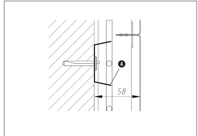
Horizontalschnitt Horizontale doorsnede
