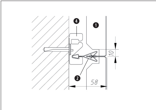
Vertikalschnitt Verticale doorsnede
