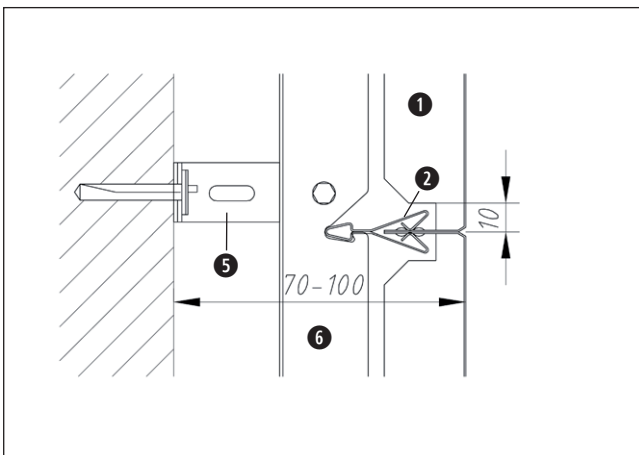
Wandverkleidung mit Modulprofil Wandbekleding met modulair muurprofiel
