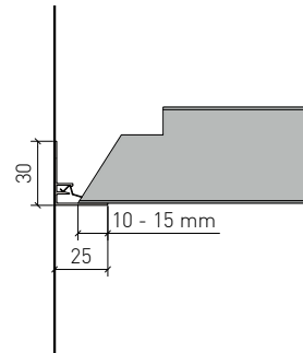
Auflage für Kassette mit Anschnitt Opleg met versneden tegel
