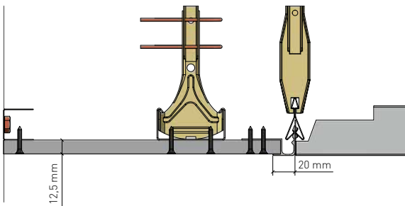
Stirnseitiger Anschluss an GK-Fries mit Übergangprofil GK (Art. Nr. 3080047 RAL 9010), Profil versetzt verschrauben. Aansluiting korte zijde paneel tegen GK-Fries met overgangprofil GK (Art. Nr. 3080047 RAL 9010), Profiel versprongen vastschroeven.
