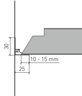
Auflage für Kassette Opleg met versneden paneel
