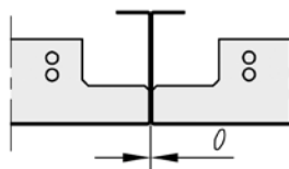
0-Fuge Senza scuretto
