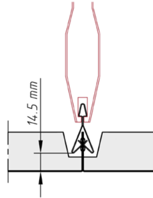
Detail B Dettaglio B
