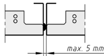
Distanzprägung Bugne distanziatrice
