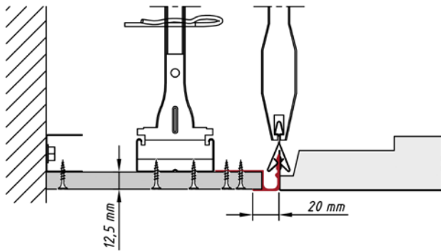
Stirnseitiger Anschluss an GK-Fries mit Übergangprofil GK, Profil versetzt verschrauben Raccord coté court avec profil GK, vissage du profil en quinconce.
