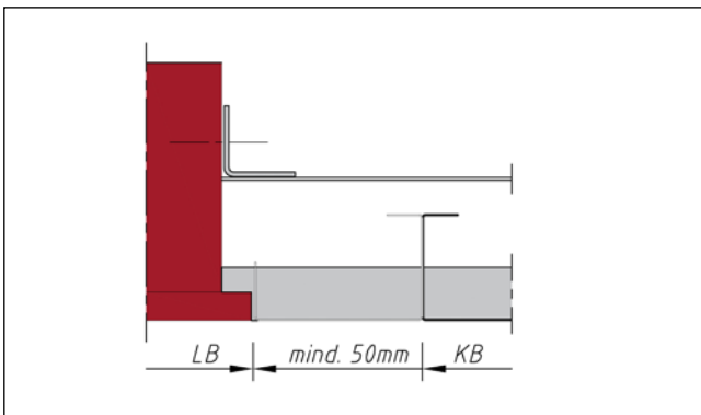
Schnitt längsseitig: Leuchte / Rostprofil Longitudinal section: light fitting / grid profile
