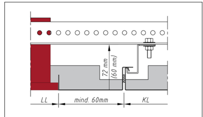
Schnitt stirnseitig: Leuchte / Rostprofil Front section: light fitting / grid profile
