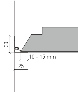
Auflage für Kassette Support for cutted tile
