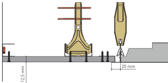
Stirnseitiger Anschluss an GK-Fries mit Übergangprofil GK (Art. Nr. 3080047 RAL 9010), Profil versetzt verschrauben. Shortside connection to gypsum frieze with gypsum connection profile (Art. Nr.3080047 RAL 9010) Profile joints on different locations to frieze joints.
