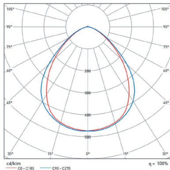
Lichtverteilung mikrop Prismatisch (BAP UGR<19) Microprismatic light distribution (BAP UGR<19)
