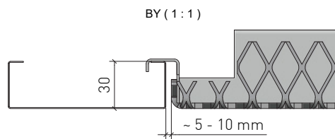
Kassettstirnseite Tile front side
