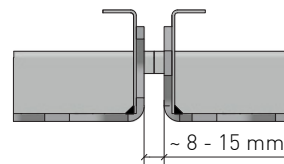
Kassettlängsseite Tile long side
