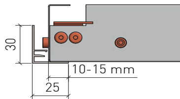
Auflage für ganze Kassette Support for entire tile
