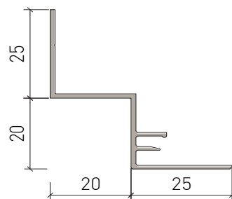
Schattenfederleiste 20/ 20 Shadow trimming section 20/ 20
