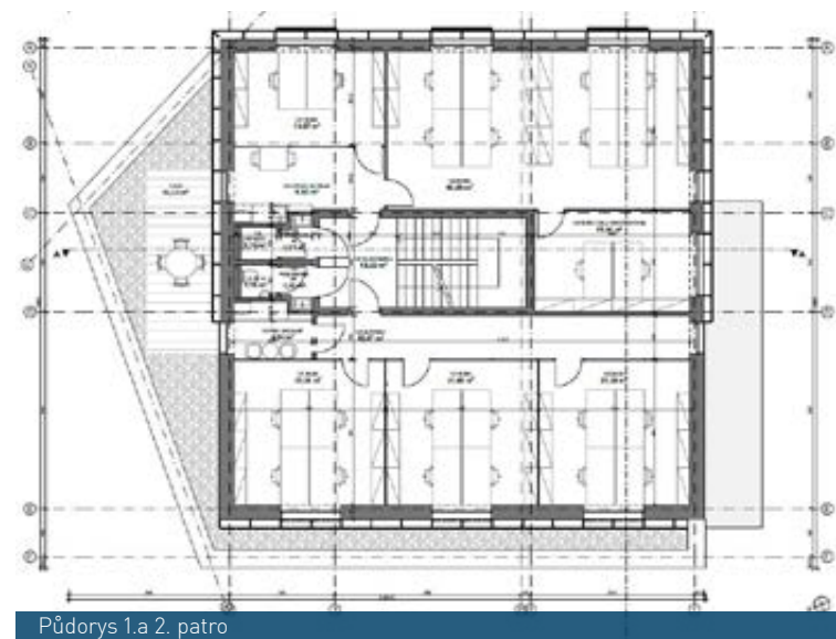
Půdorys 1.a 2. patro
