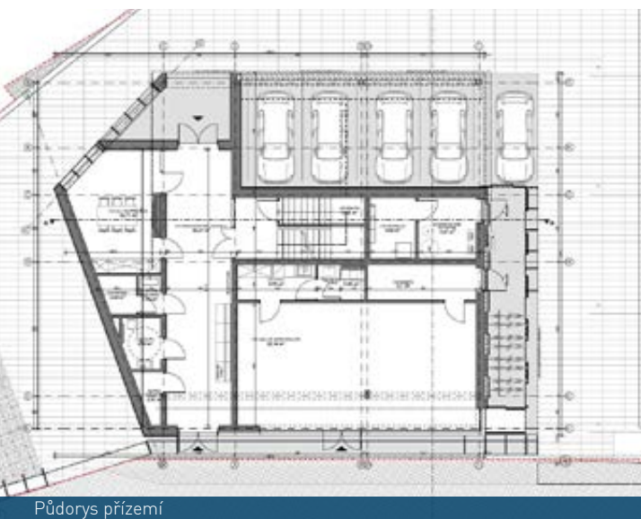
Půdorys přízemí
