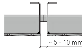
Kassettenlängsseite Tile long side
