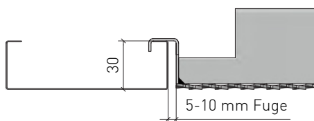
Kassettenstirnseite Tile front side
