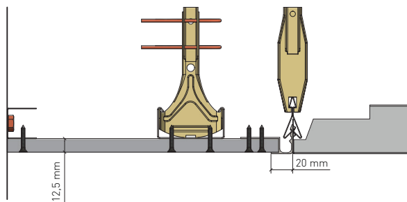
Stirnseitiger Anschluss an GK-Fries mit Übergangsprofil GK (Art. Nr. 3080047 RAL 9010), Profil versetzt verschrauben. Připojení k sádrokartonu pomocí přechodového profilu GK (výr.č. 3080047 RAL 9010), profil šroubovat odsazeně
