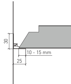
Auflage für Kassette Položení řezané kazety
