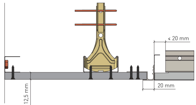
Stirnseitiger Anschluss an GK-Fries, Profil versetzt verschrauben
