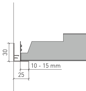
Auflage für ganze Kassette Položení celé kazety
