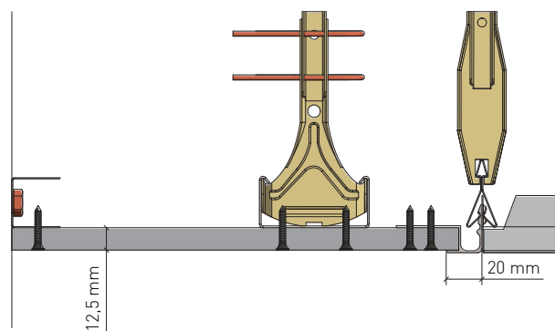
Stirnseitiger Anschluss an GK-Fries mit Übergangsprofil GK (Art. Nr. 3080047 RAL 9010), Profil versetzt verschrauben.
