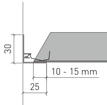
Auflage für Kassette mit Anschnitt Položení řezané kazety
