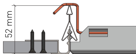
Anschluss Gipskartonfries mit Übergangsprofil GK-Fries (3080047, RAL 9010) Připojení na sádrokarton (3080047, RAL 9010)
