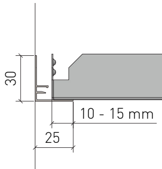
Auflage für ganze Kassette Položení celé kazety
